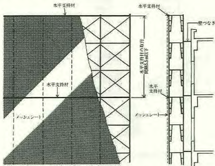
鋼管足場への設置例
