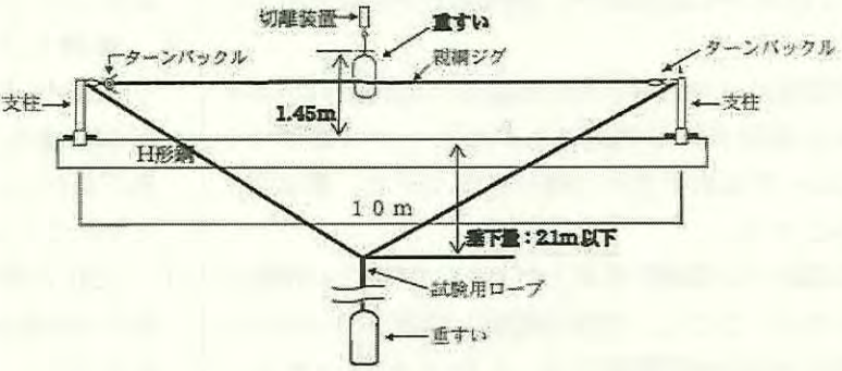
落下阻止性能試験の例（平行型）
