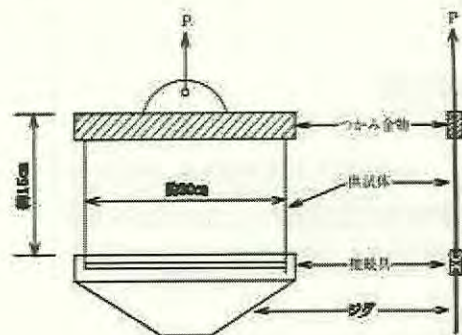
接続具の引き抜き試験の例
