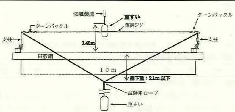
落下阻止性能試験の例（直交型）
